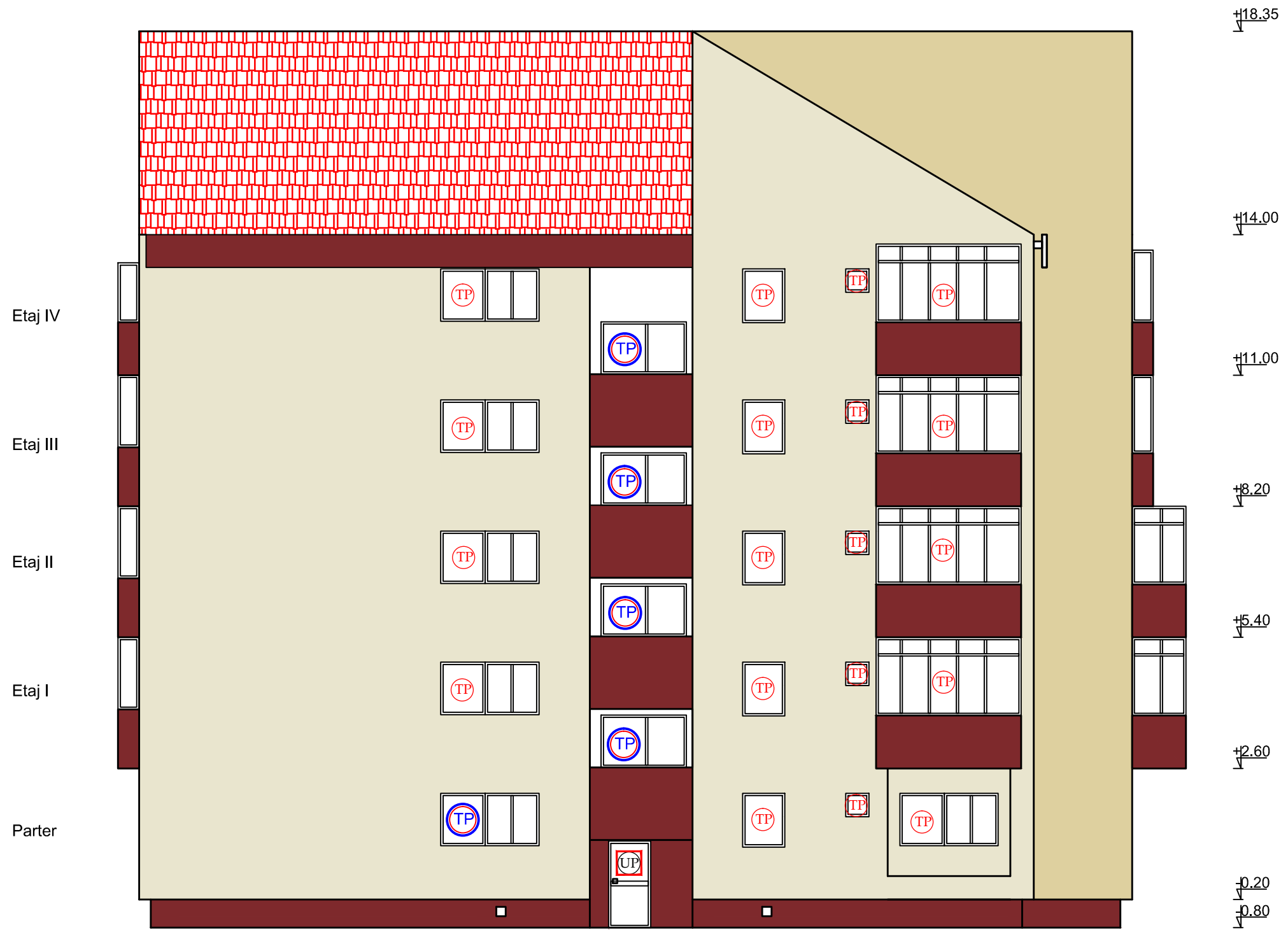
Fatada posterioara propusa Scara 1:100
